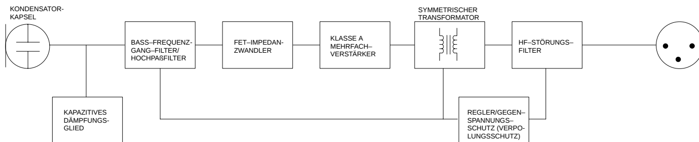
BLOCKSCHALTBILD ABBILDUNG 6
