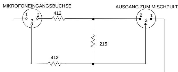
15-DB-DÄMPFUNGSGLIED-SCHALTUNG ABBILDUNG 5
