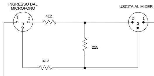
CIRCUITO ATTENUATORE DA 15 DB FIGURA 5
