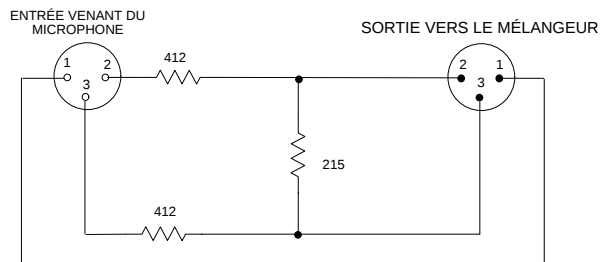
CIRCUIT ATTENUATEUR 15 DB
