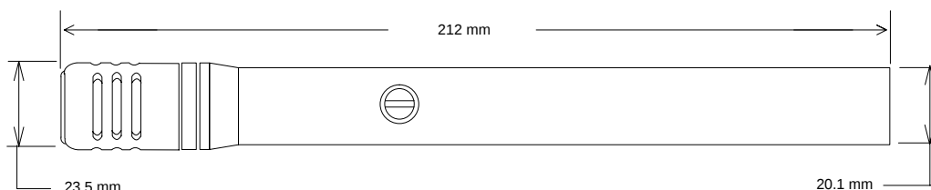
DIMENSIONES GENERALES FIGURA 3
