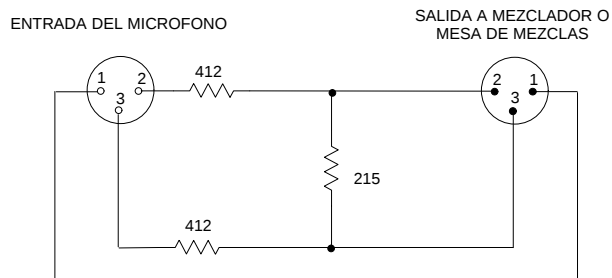
CIRCUITO ATENUADOR DE 15 DB
