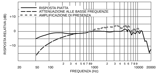
RISPOSTA IN FREQUENZA TIPICA FIGURA 1
