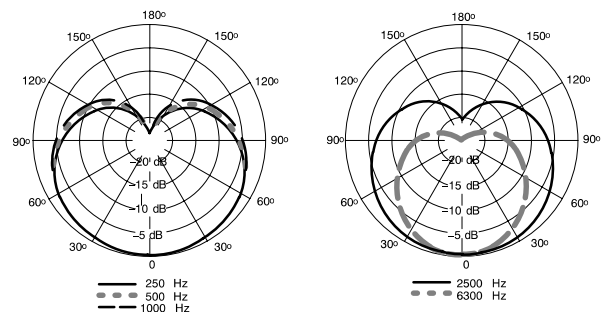
TYPISCHE RICHTCHARAKTERISTIKEN
