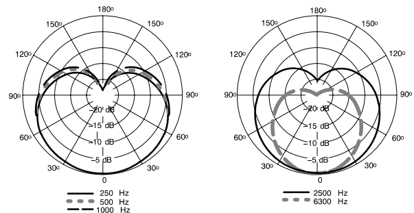
DIAGRAMMI POLARI TIPICI FIGURA 2
