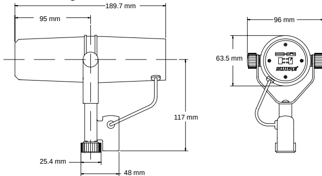
DIMENSIONES GENERALES
