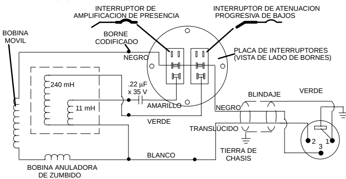
CONEXIONES INTERNAS
